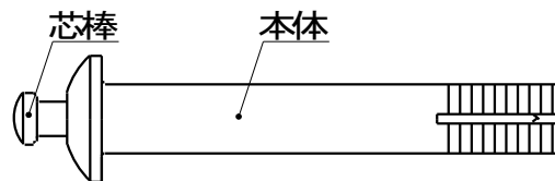
ハイアンカー ST タイプの部品構成
