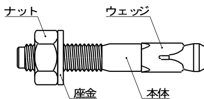
ハイアンカーHW タイプの部品構成 (HW3068TN 除く)
