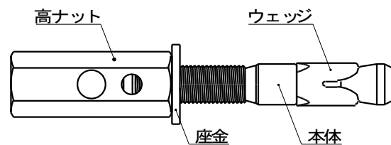
ハイアンカーHW3068TN の部品構成
